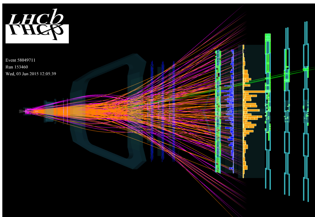
Rysunek 1. Przykład typowego przypadku oddziaływania proton-proton przy energii LHC. Linie reprezentują zrekonstruowane trajektorie cząstek powstałych w oddziaływaniu.
