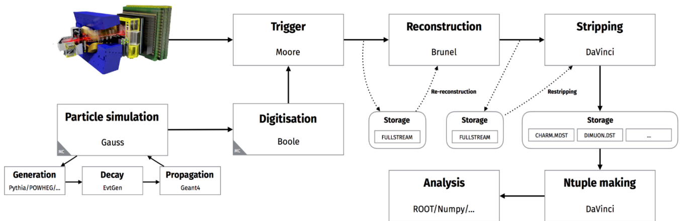
Rysunek 5. Schemat przetwarzania danych (symulowanych oraz 'prawdziwych') dla eksperymentu LHCb.
